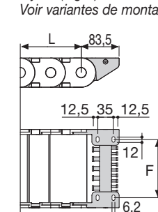
Fig. B Fixation standard extérieure au rayon. (Fig B) Voir variantes de montage page 31.
