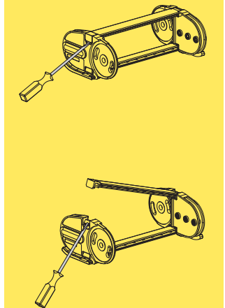
Séparation horizontale Pour le choix des séparateurs voir page. 216
