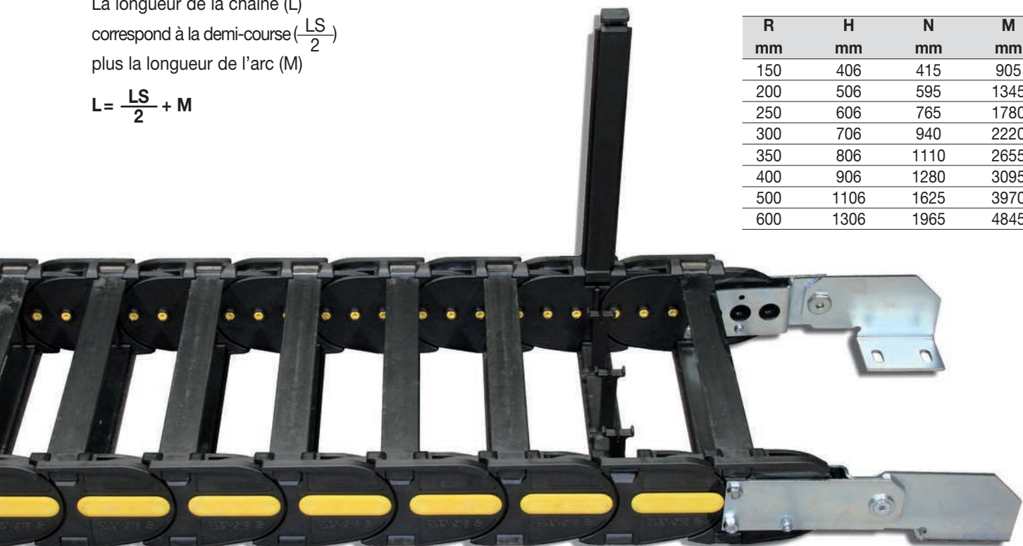
Version avec entretoises assemblés tous les pas
