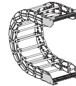
图B 拖链是通过弯曲段的外侧进行固定的。见第31页端部接头的各种安装方式
