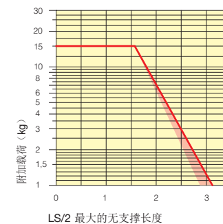
LS/2 最大的无支撑长度
