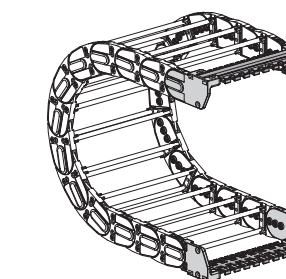
图B 拖链是通过弯曲段的外侧进行固定的。见第31页端部接头的各种安装方式
